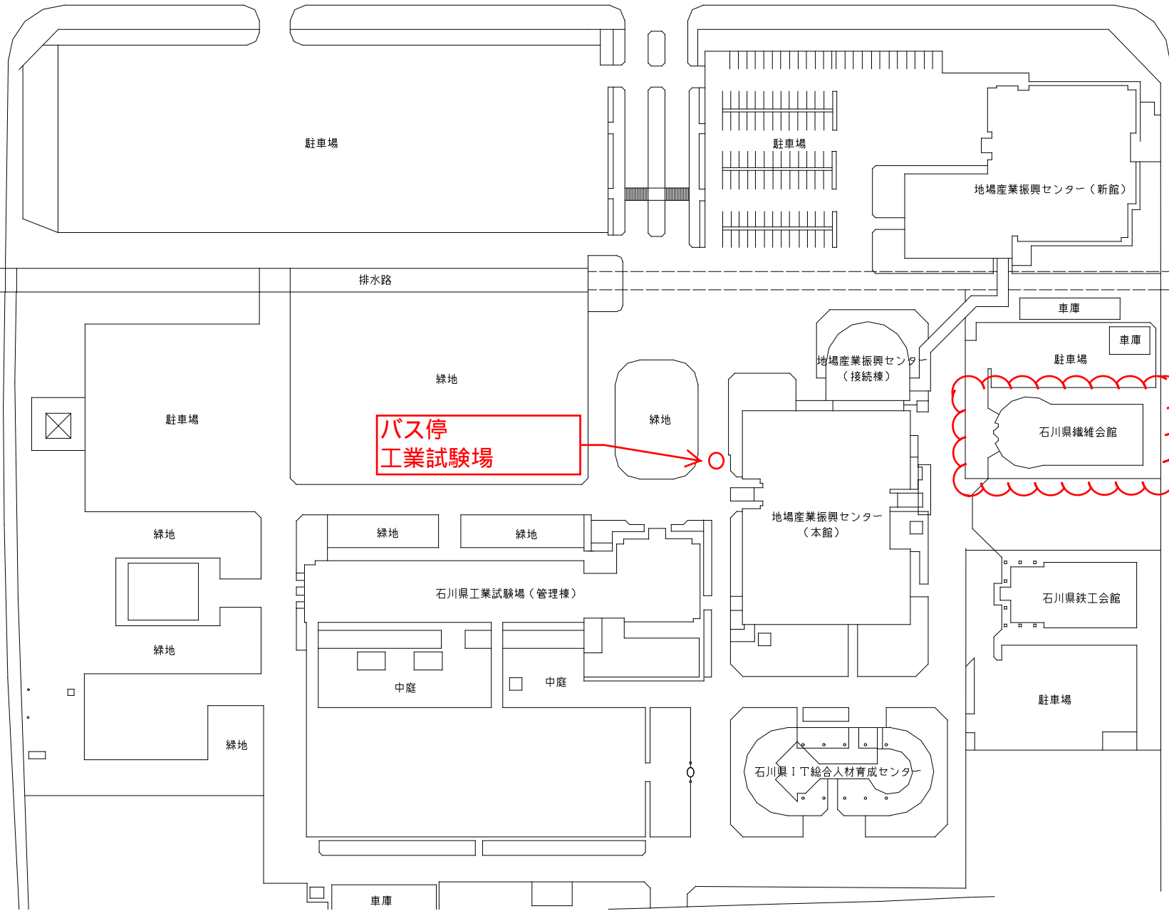
地場産業センター敷地平面図
